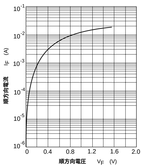
図1. 順方向特性
