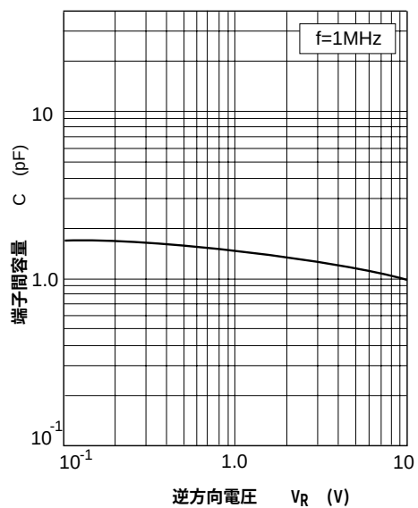
図3. 端子間容量 対 逆電圧特性
