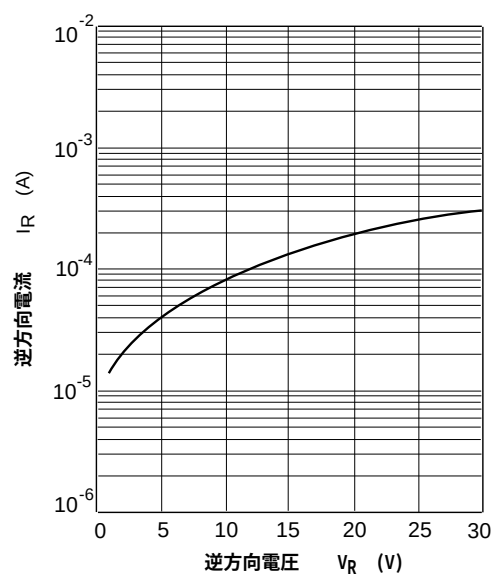
図2. 逆方向特性
